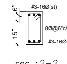
sec : 2-2
