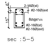
sec : 5-5
