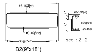
B2(9"x18")
