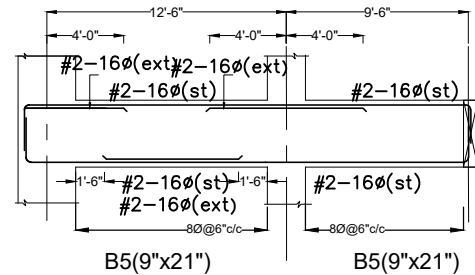
B5(9"x21") B5(9"x21")
