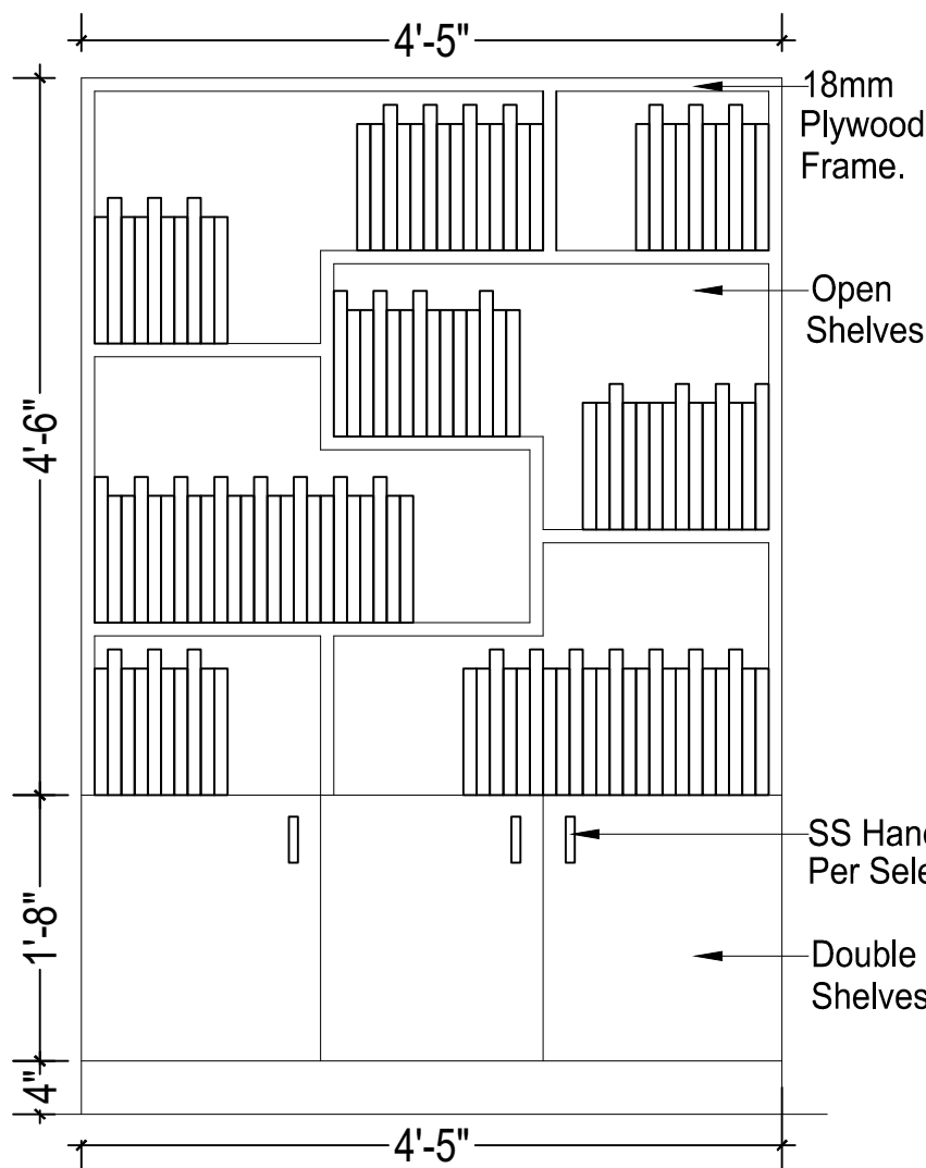
ELEVATION
