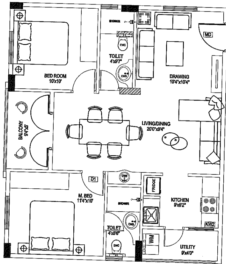
TYPE - B
