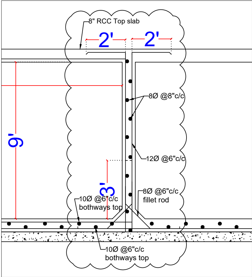
Detail-B
