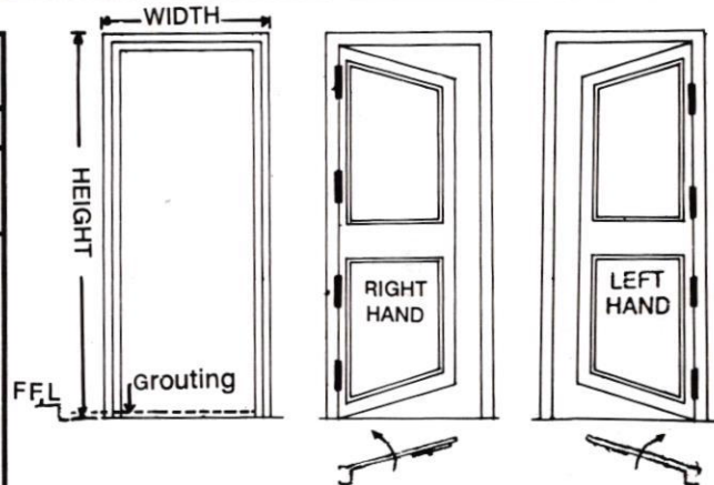
DOOR FRAME & SHUTTER
