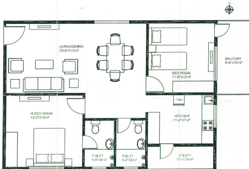
TYPE - VI 1220 SFT
