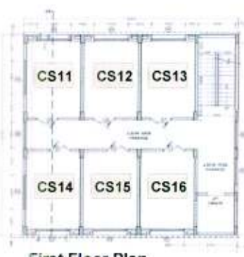
First Floor Plan (Scale – N.T.S.)
