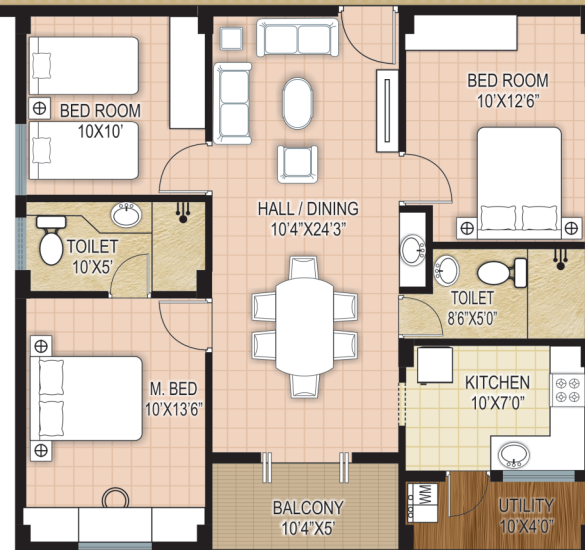
TYPE : C - 1210 sft.
