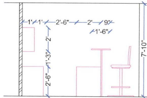
SECTION-A
