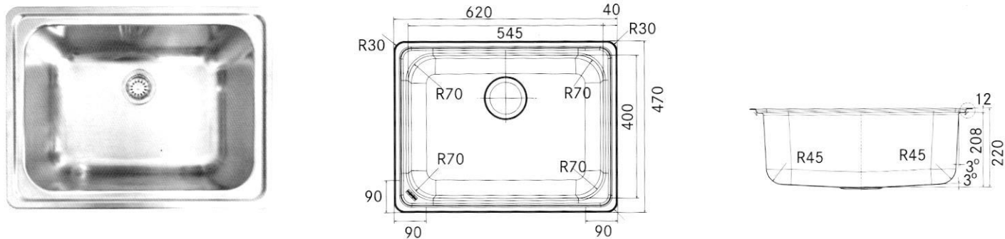
RSX 6 10-63 (24"x18")
