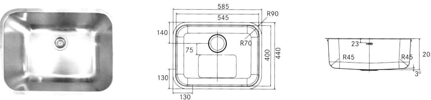
RSX 2 10-55 (23"x18")
