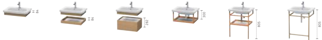
Wash basin panel ↔ 580 ↗ 448 # DS 6080 ↔ 730 ↗ 448 # DS 6081 ↔ 930 ↗ 448 # DS 6082 ↔ 1130 ↗ 448 # DS 6083 Storage board ↔ 580 ↗ 448 # DS 6181 ↔ 730 ↗ 448 # DS 6182 ↔ 930 ↗ 448 # DS 6183 # ↔ 1130 ↗ 448 DS 61834 Low cabinet ↔ 580 ↗ 448 # DS 6280 ↔ 730 ↗ 448 # DS 6281 ↔ 930 ↗ 448 # DS 6282 ↔ 1130 ↗ 448 # DS 6283 Storage board ↔ 590 ↗ 440 # DS 9871 ↔ 740 ↗ 440 # DS 9872 ↔ 940 ↗ 440 # DS 9873 ↔ 1140 ↗ 440 # DS 9874 Towel rail with storage board ↔ 590 ↗ 440 # DS 9881 ↔ 740 ↗ 440 # DS 9882 ↔ 940 ↗ 440 # DS 9883 ↔ 1140 ↗ 440 # DS 9884 Towel rail ↔ 590 ↗ 440 # DS 9891 ↔ 740 ↗ 440 # DS 9892 ↔ 940 ↗ 440 # DS 9893 ↔ 1140 ↗ 440 # DS 9894
